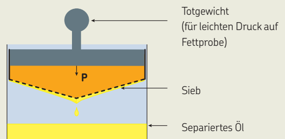
Ölabscheidungstest
