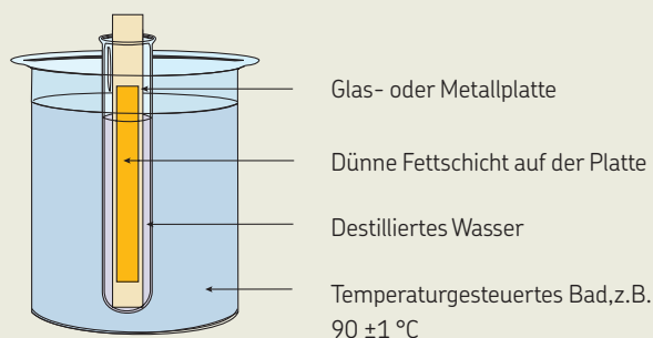
Test - Verhalten gegenüber Wasser
