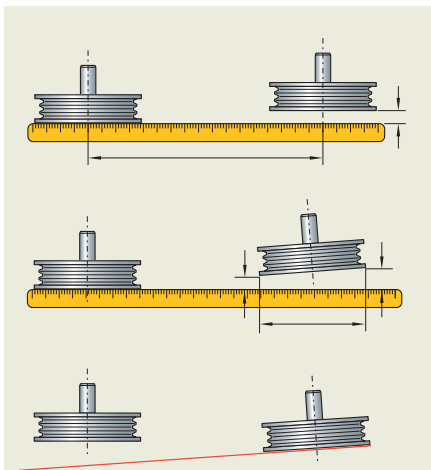
Messung des Parallel- und Winkerversatzes mit Hilfe eines Lineals oder einer Schnur.
